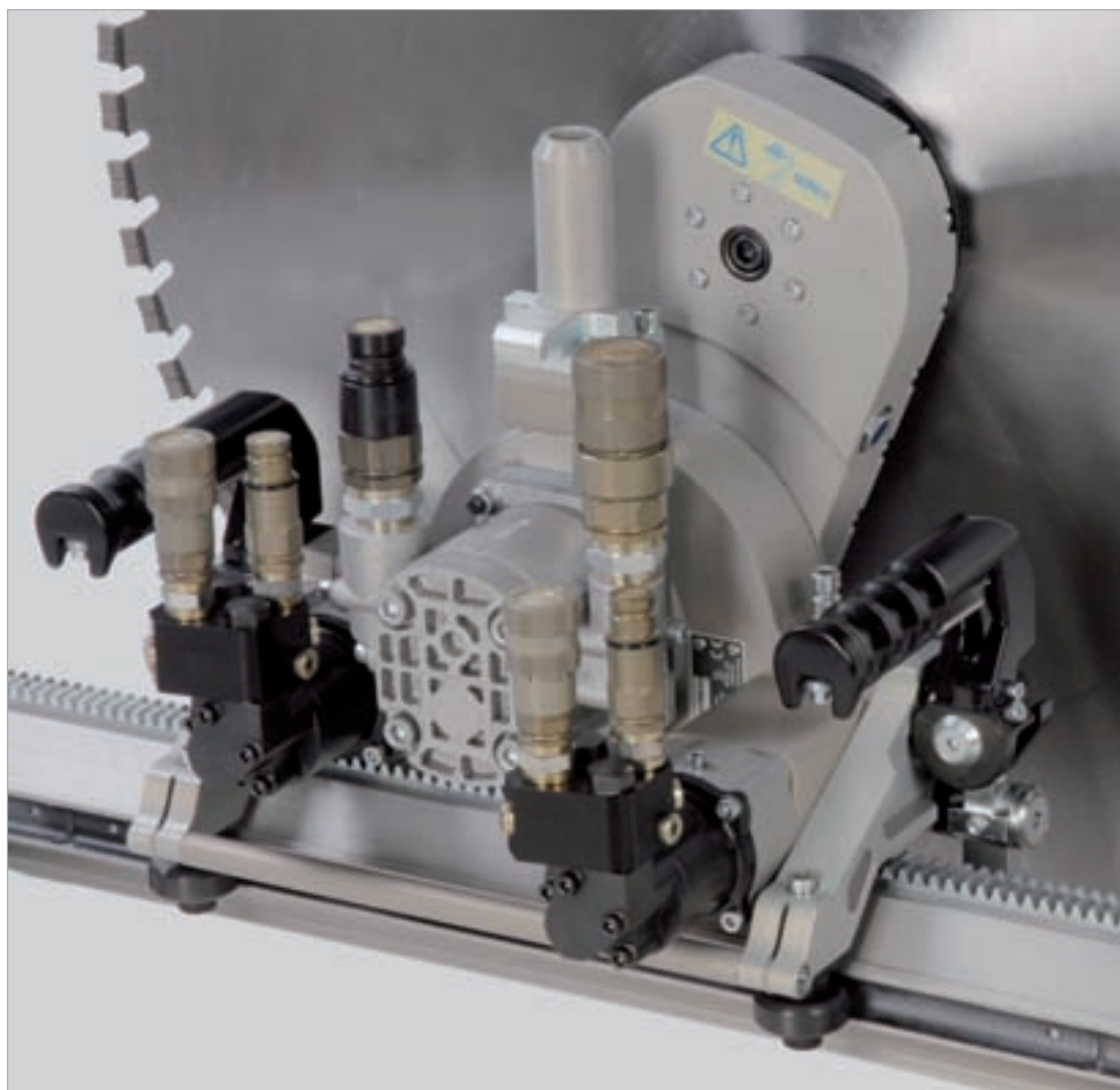
Veggsaghode av høyfast aluminiumslegering, tannhjuls-svingarm og rulleføringer
