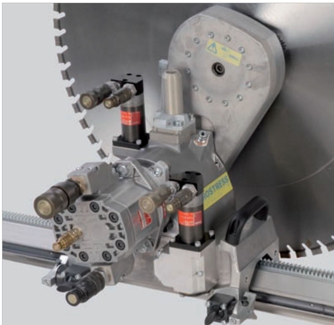
Hovedmotor med lekkoljettkobling
